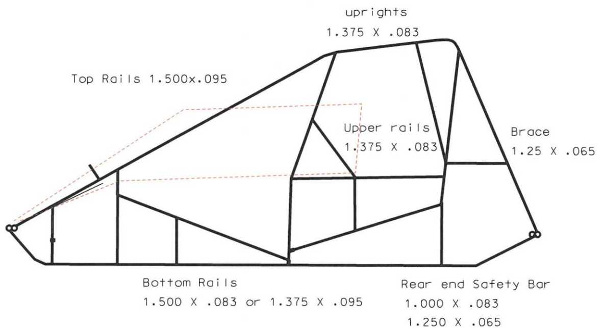
Roll Cage
